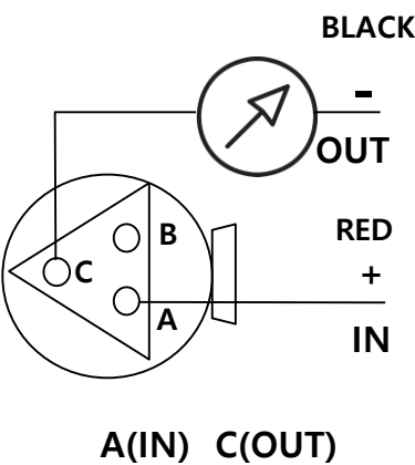
Deutsch DT04-03P
