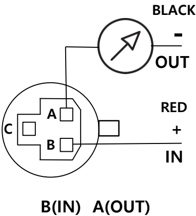
Packard
