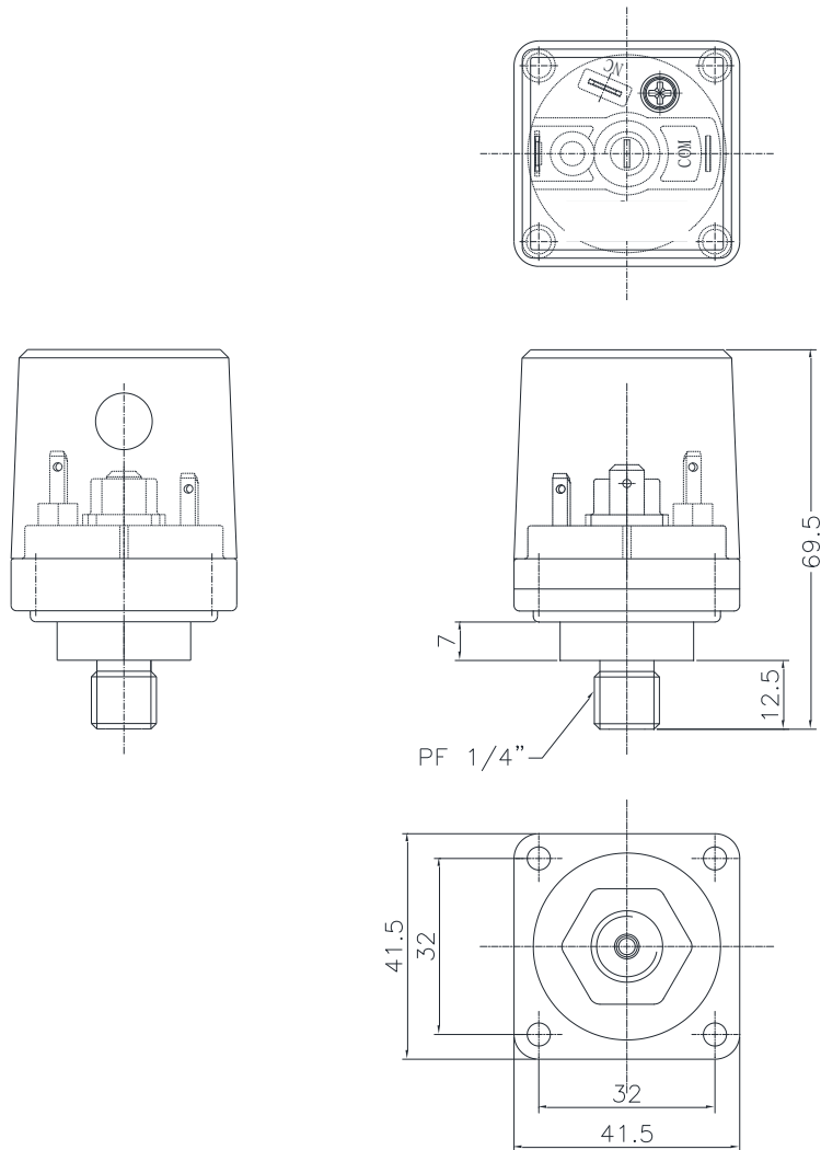
Fig 1. 가스압스위치(고정형)
